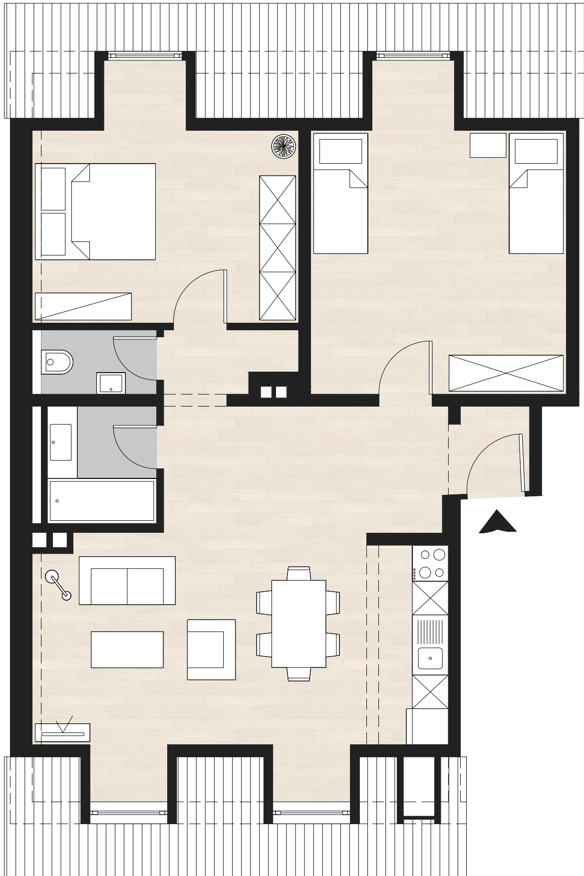
Wohnung links
